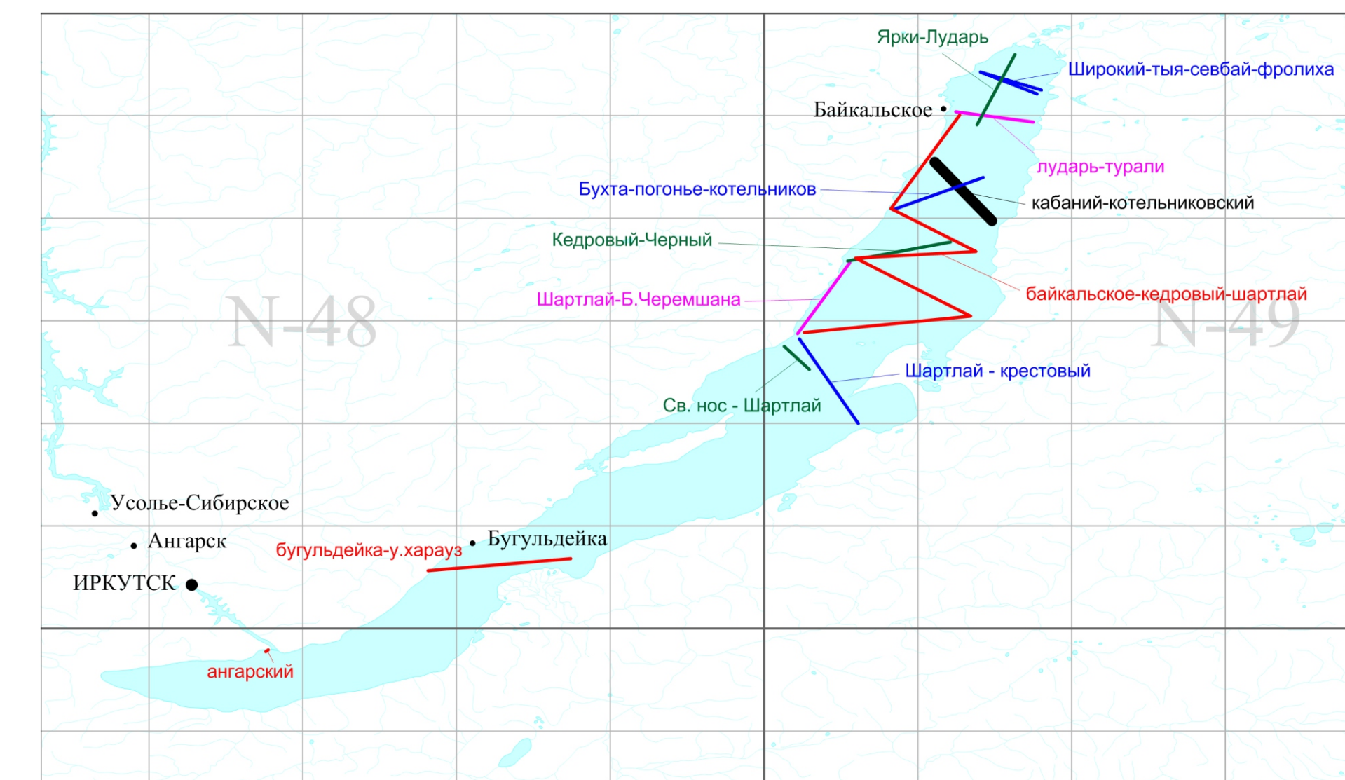
Непрерывное сейсмоакустическое профилирование (НСП) на Байкале Исходный разрез по профилю "Кабаний-котельниковский" Наблюдение 1992-93 гг. Ларкин Г.В. Составили: Гриценко С.А., Зайцев С.А.
