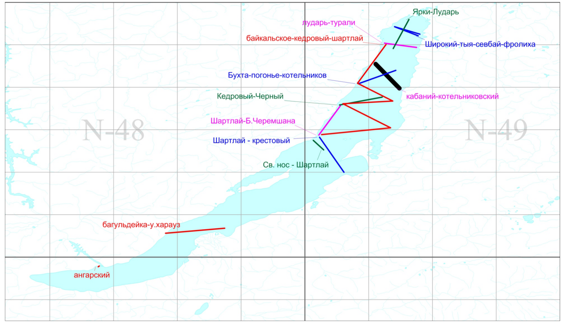
Непрерывное сейсмоакустическое профилирование (НСП) на Байкале Цветовое изображение (метод RGB) временного разреза по профилю "Кабаний-котельниковский", обработанного в системе CubeTechnology в лаборатории "Методических разработок обработки и интерпретации сейсмических данных" ФГУП ВСЕГЕИ - 2015г.
