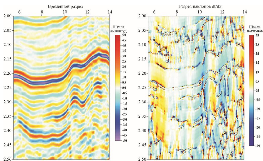
Рис. 6.2. Временной разрез и его наклоны
