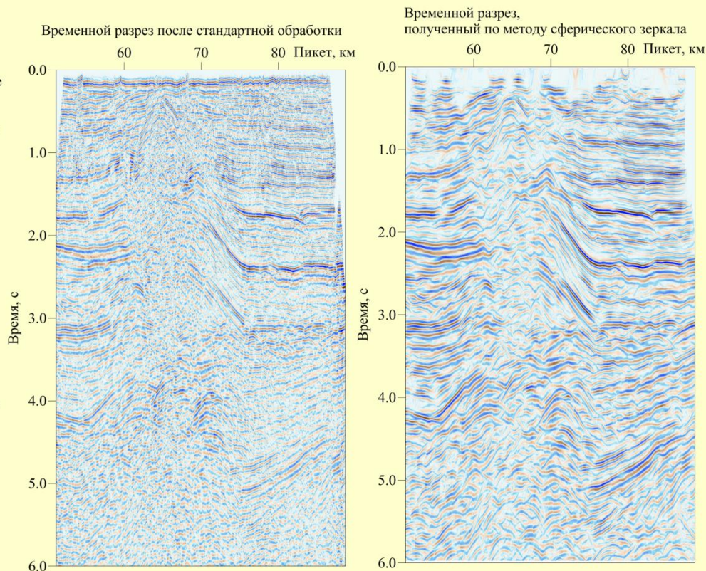
Метод сферического зеркала
