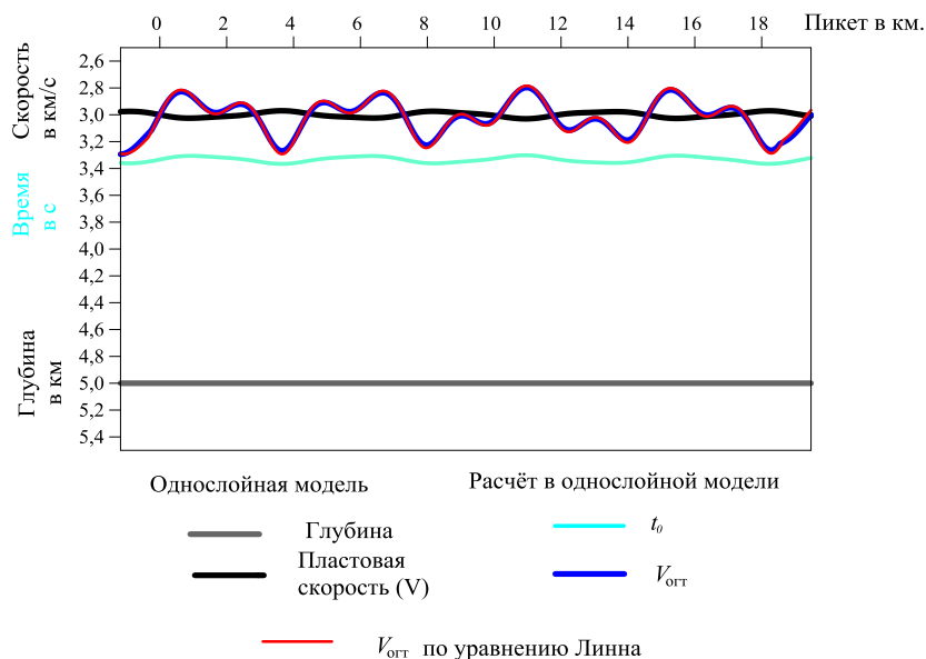
Рис. 4.2. Проверка уравнения Линна
