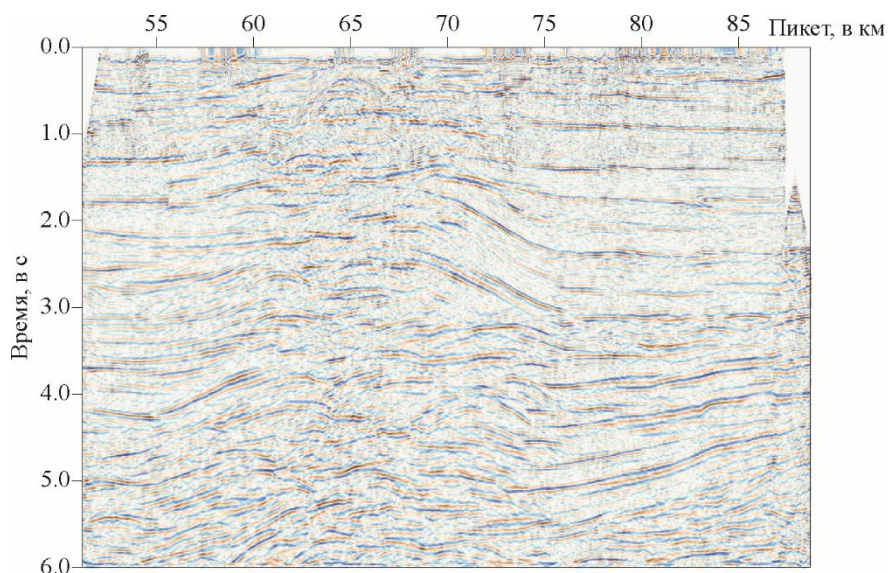
Рис. 3.10. Временной разрез после КФ
