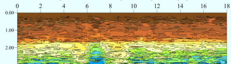
Влияние зоны растепления вечной мерзлоты на временной разрез скоростей суммирования
