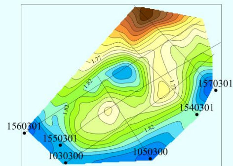
Структурная карта в районах проявления вечной мерзлоты
