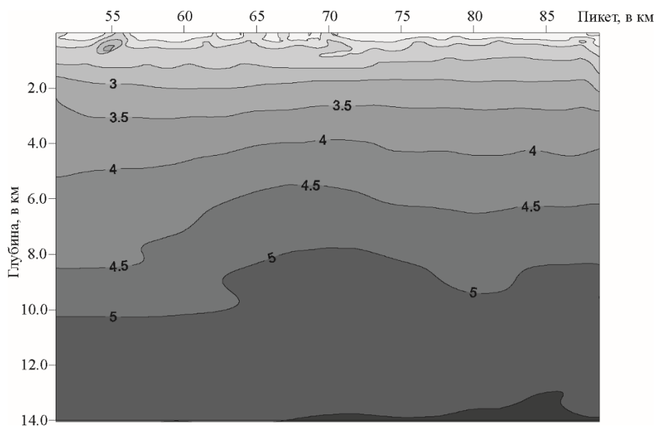
Рис. 4.7. Глубинный разрез средних скоростей
