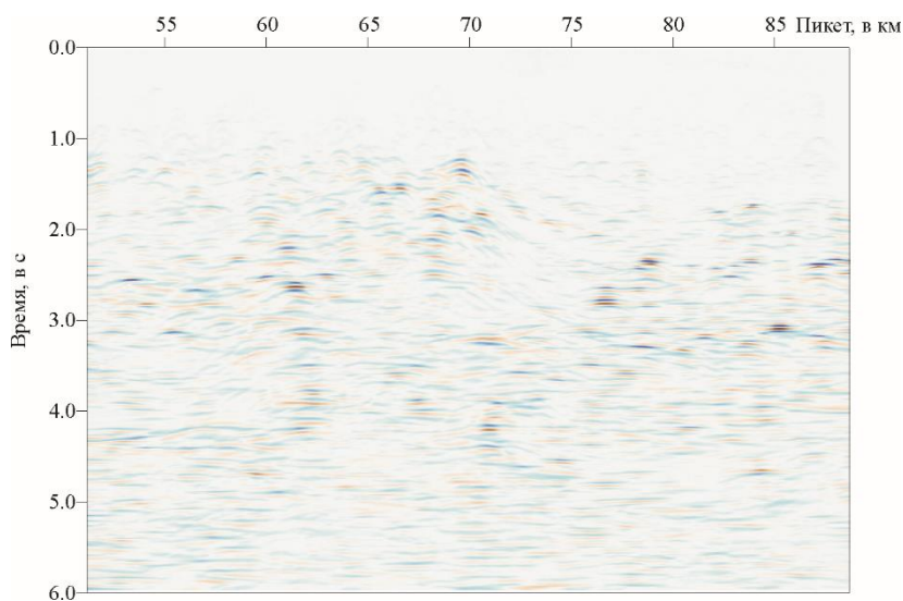
Рис. 5.4. Миграция Кирхгофа разреза дифрагированных волн
