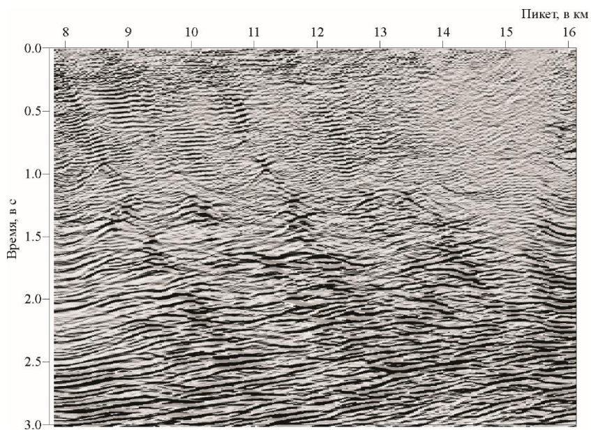
Рис. 5.7. Мексиканский залив. Миграция Кирхгофа разреза дифракции
