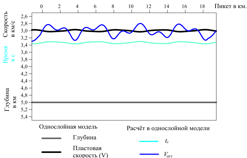
Рис. 3.1. Расчёт в однослойной модели с горизонтальной отражающей границей на глубине 5 км и латеральным изменением пластовой скорости V = 3 + 0,025\sin(1,3X) + 0,005*\sin(3X)
