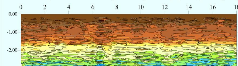
Коррекция временного разреза скоростей суммирования в зоне растепления
