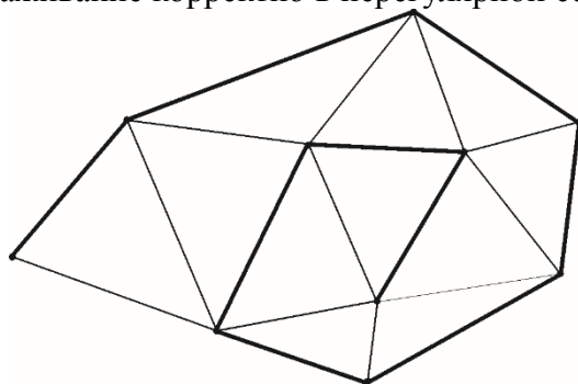
Рис. 6.7. Триангуляция Делоне
