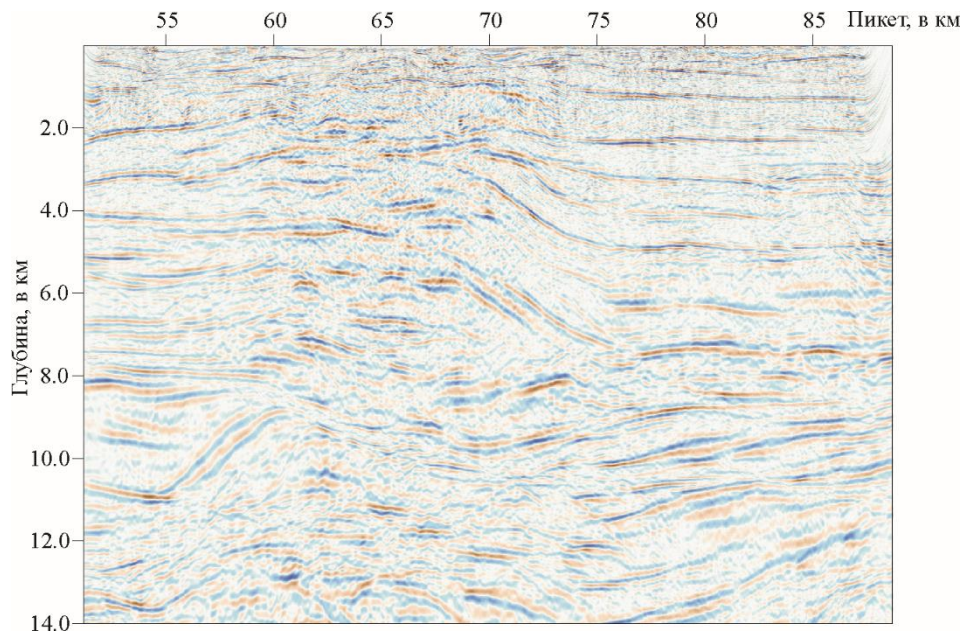
Рис. 4.8. Глубинный мигрированный разрез
