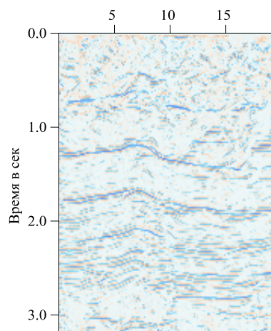
Обработка методом «сферического зеркала»
