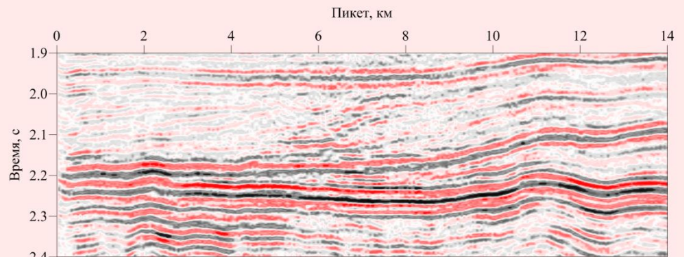
Временной разрез
