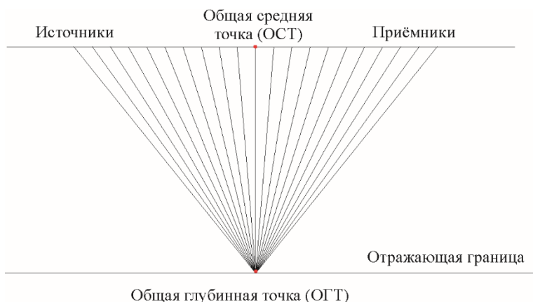
Рис. 1.2. Зеркальное отражение в ОГТ
