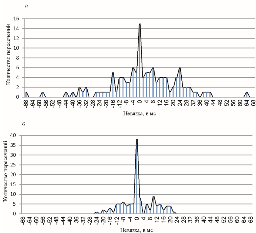
Рис. 6.3. Гистограммы невязок (а – до и б – после минимизации)
