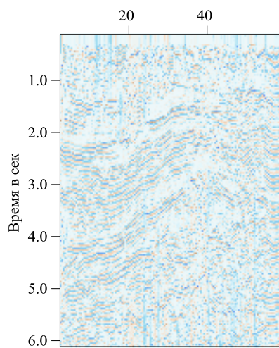
Обработка методом «сферического зеркала»
