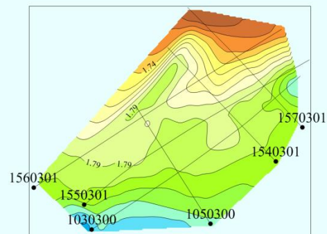
Та же структурная карта после коррекции в зонах неоднородностей вечной мерзлоты
