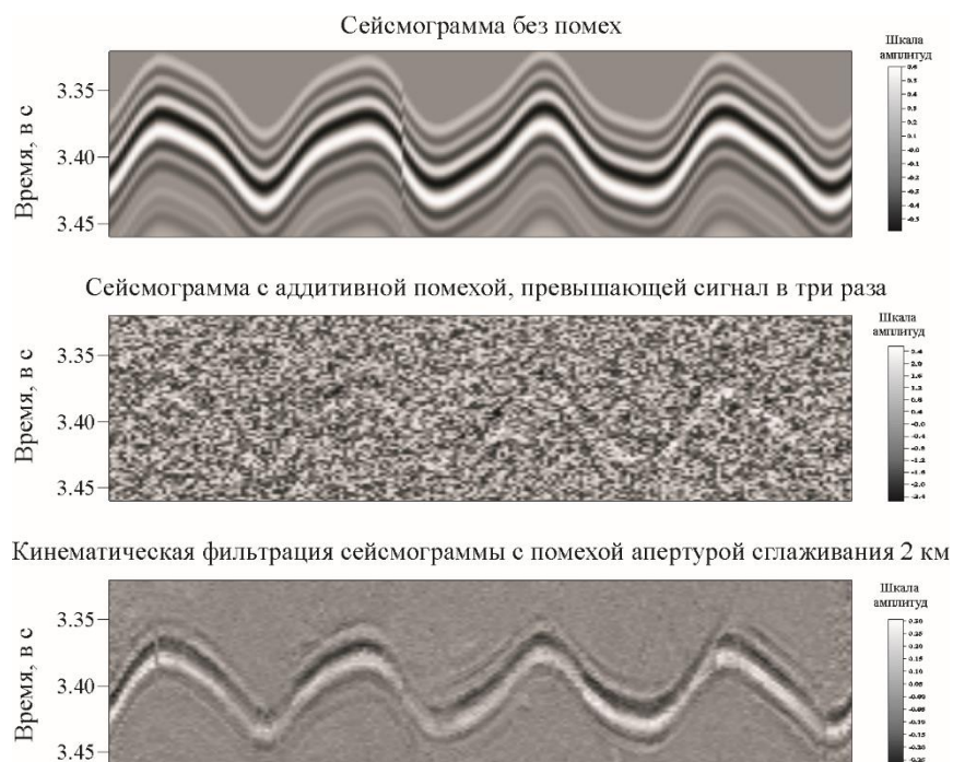
Рис. 3.3. Сейсмограммы общих удалений для расстояния 900 м источник-приёмник
