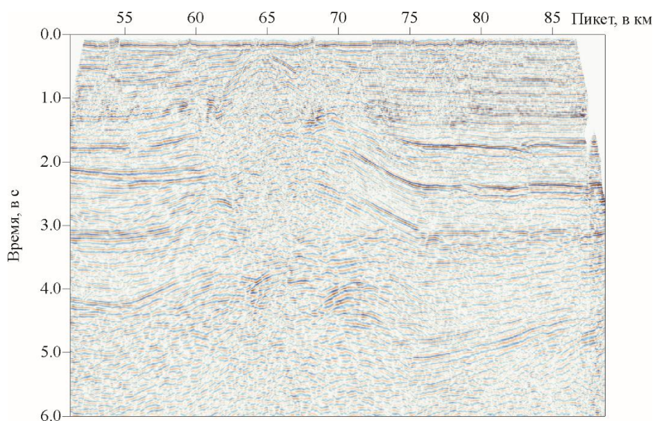
Рис. 3.7. Временной разрез
