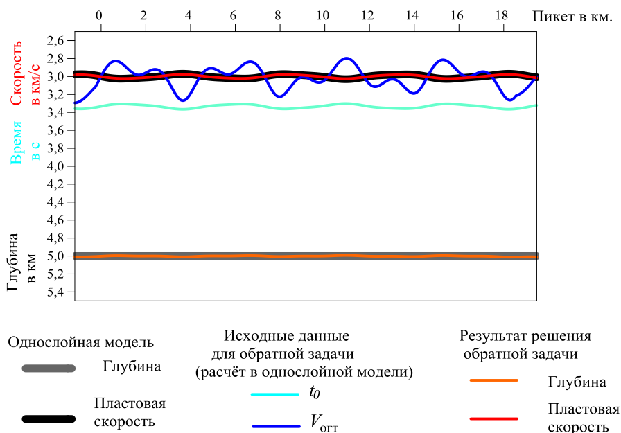
Рис. 4.3. Решение обратной задачи в однослойной модели с латеральным изменением пластовой скорости
