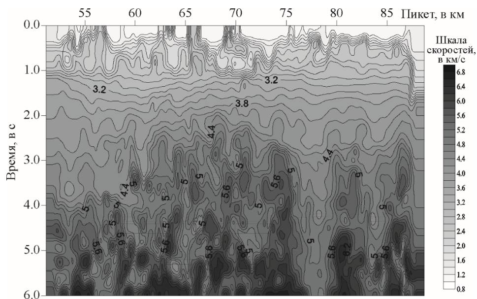
Рис. 3.9. Временной разрез скоростей суммирования
