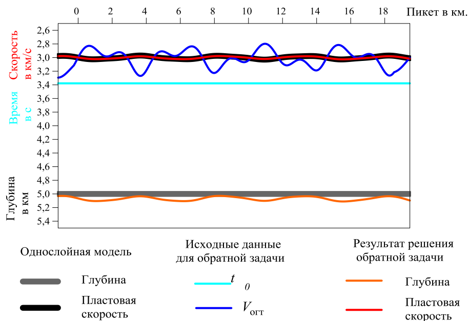
Рис. 4.4. Решение обратной задачи в однослойной модели с постоянным значением t_0
