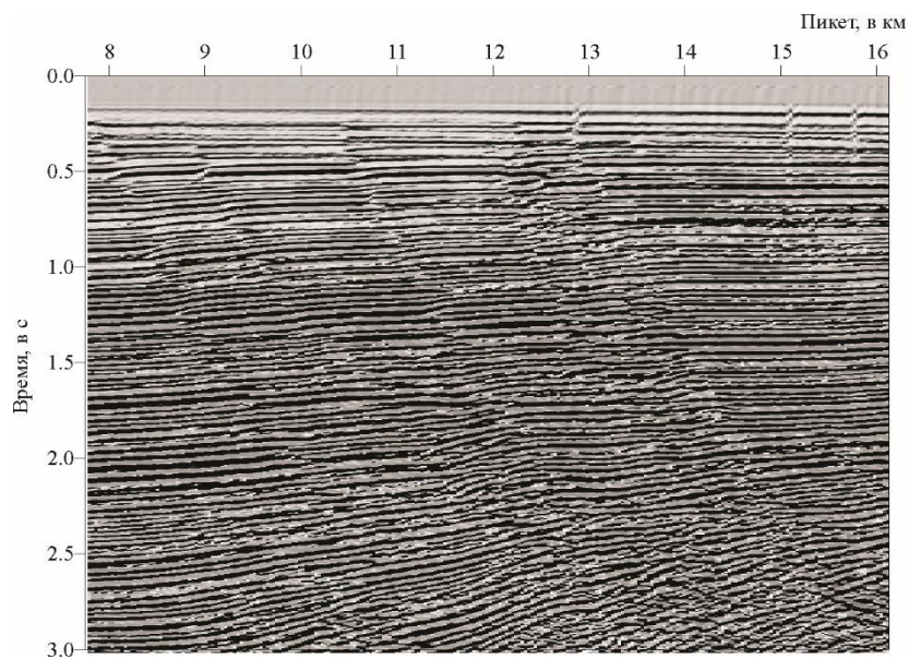
Рис. 5.5. Мексиканский залив. Исходный временной разрез
