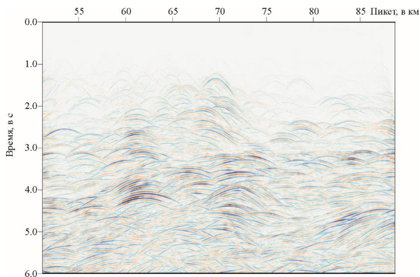
Рис. 5.3. Хатангский залив. Разрез дифрагированных волн
