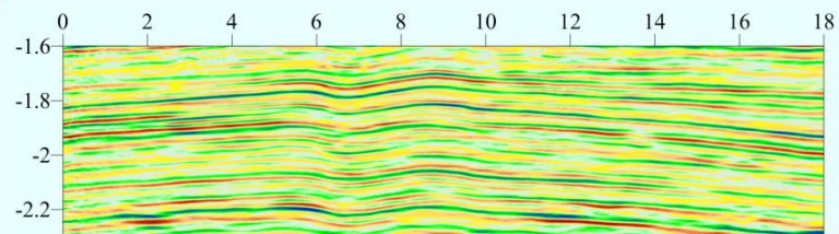
Влияние зоны растепления вечной мерзлоты на временной разрез
