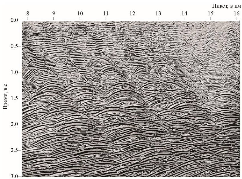
Рис. 5.6. Мексиканский залив. Разрез дифракции
