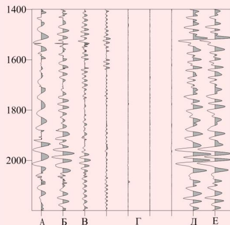
Экспоненциальное разложение трассы временного разреза
