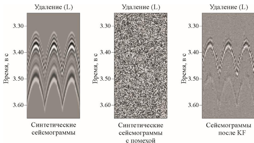
Рис. 3.4. Сейсмограммы ОГТ
