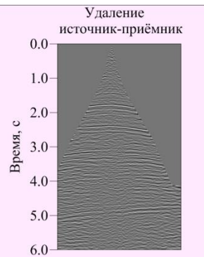
Сейсмограмма ОТВ после стандартной обработки
