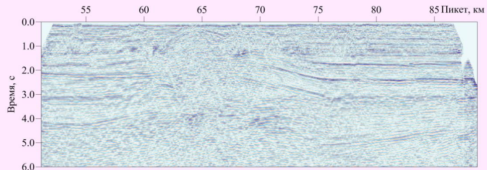
Временной разрез после стандартной обработки (акватория моря Лаптевых, Хатангский залив)
