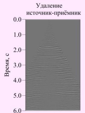
Сейсмограмма ОТВ после кинематической фильтрации
