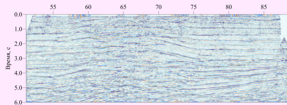
Временной разрез, полученный по сейсмограммам после кинематической фильтрации
