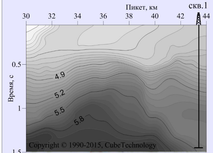
Разрез скоростей рассчитанный по разрезу дифракции
