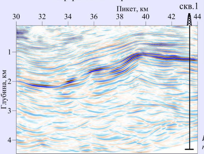
Глубинный разрез, построенный путем миграции с использованием разреза скоростей
