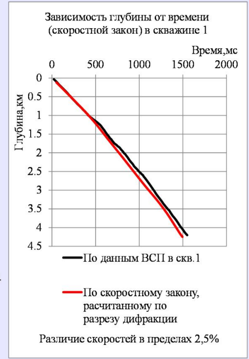
Сравнение скоростных законов по данным ВСП и скоростному разрезу в скв. 1
