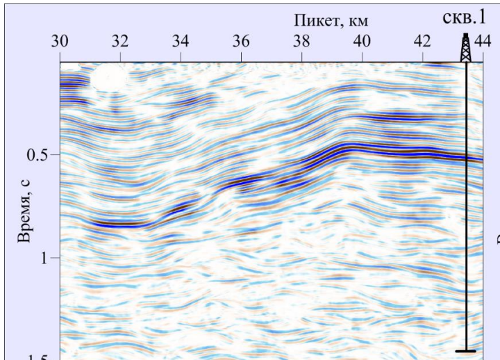
Исходный временной разрез
