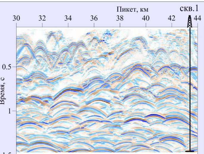
Разрез дифракции, построенный по методу "сферического зеркала"
