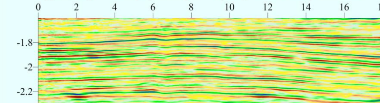
Коррекция временного разреза в зоне растепления
