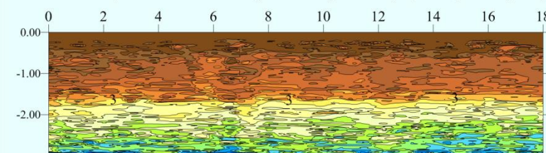
Коррекция временного разреза скоростей суммирования в зоне растепления
